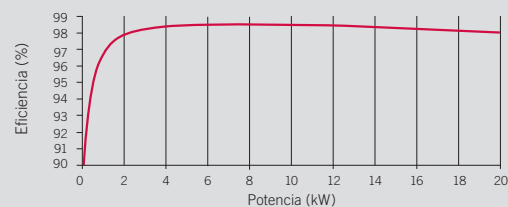
Rendimiento INGECON® SUN 20TL V_{dc} = 600 V
